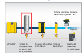
Instalación antes del sistema de tratamiento del aire comprimido
