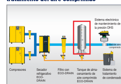
Instalación después del sistema de tratamiento del aire comprimido
