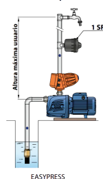
Instalación típica
